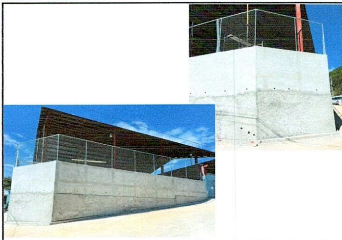
Foto 1: Finalización del muro de contención, en las fotografías se puede observar la construcción en la parte exterior.
